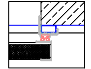
DETAY E
